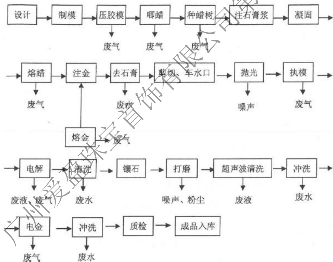
工艺流程 1
