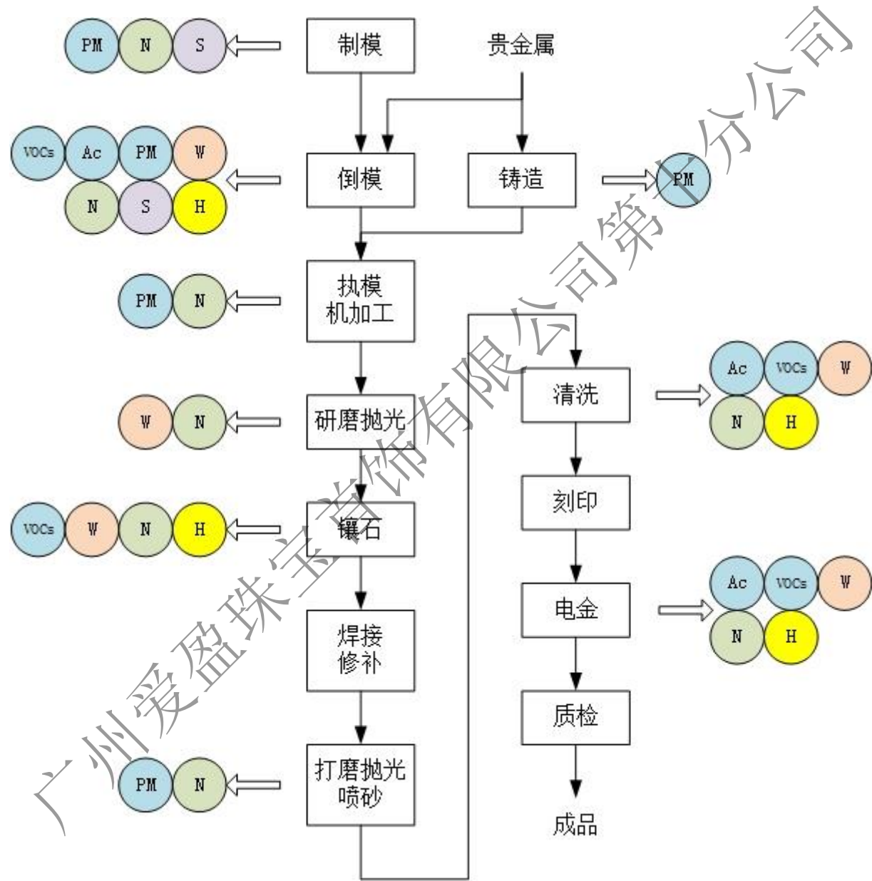
图 2 工艺流程和产污环节示意图
