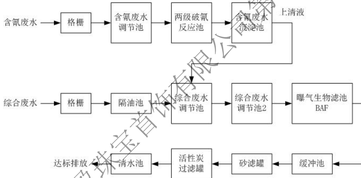
图 4 加工区废水处理站工艺流程图
