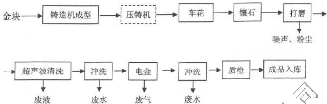
工艺流程 2
