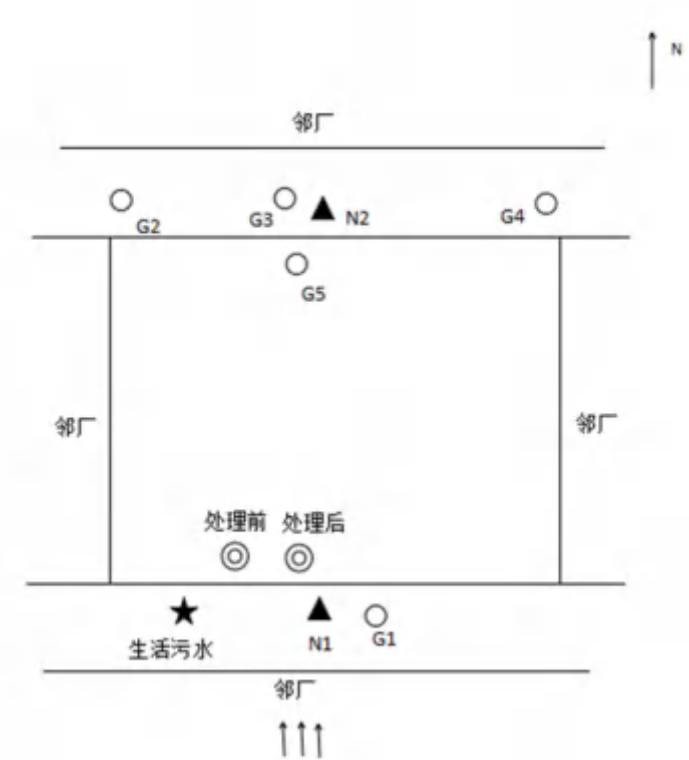
图 7-1 项目废水、废气及噪声监测点位示意图
