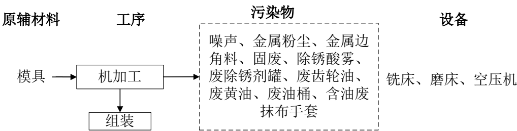
图 3-2 模具制造生产工艺流程图
