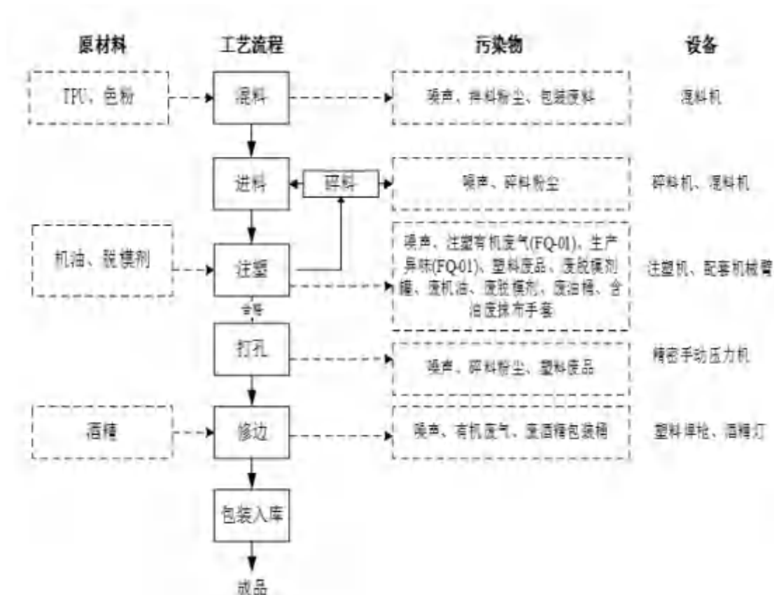
图 3-1 项目生产工艺流程及产污环节示意图
