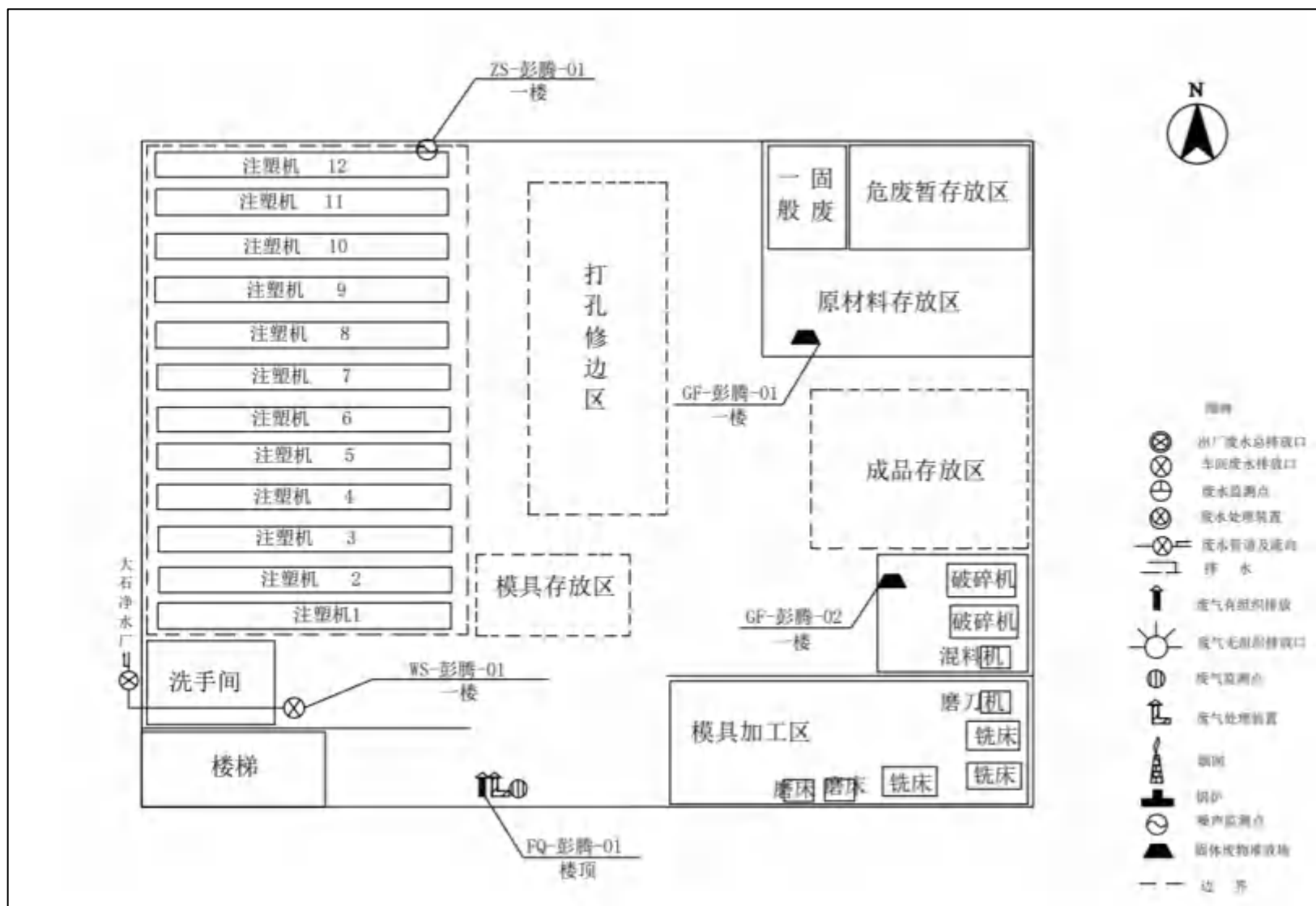
图3-4 项目排污点位图
